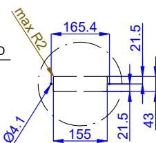
Dettaglio □ Scala 1:7
